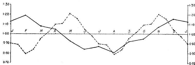
Tokio (MILNE).
